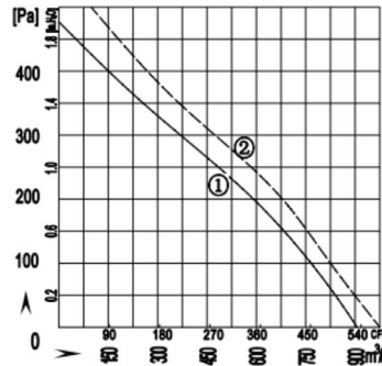
■ P-Q曲线 P-Q Curve
