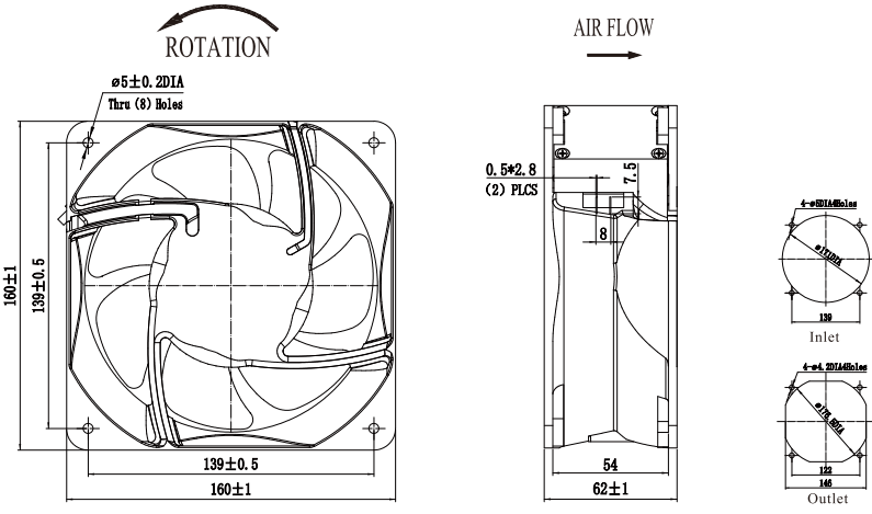
■ 外观尺寸 (mm) Dimensions (mm)
