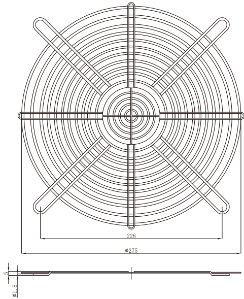
▪ JL-250 For 250mm Fan
