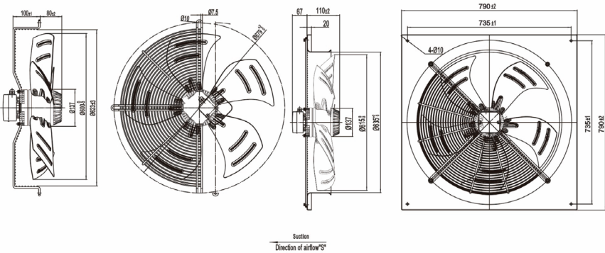
外观尺寸 (mm) Dimensions (mm)
