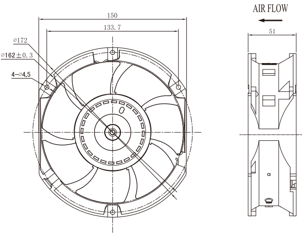
外观尺寸 (mm) Dimensions (mm)
