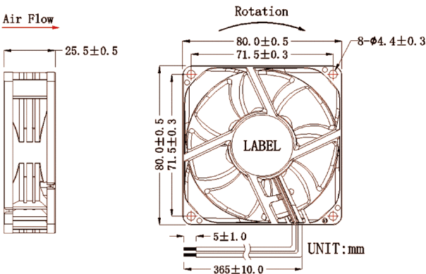
外观尺寸 (mm) Dimensions (mm)
