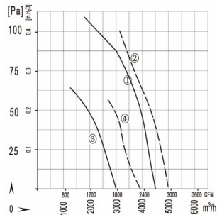
■ P-Q曲线 P-Q Curve
