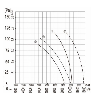
P-Q曲线 P-Q Curve
