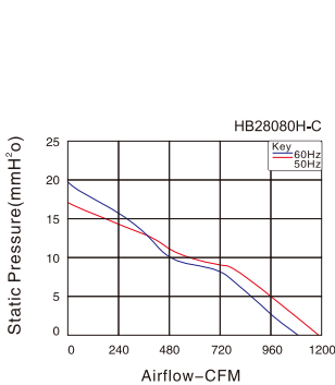
■ P-Q曲线 P-Q Curve
