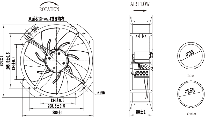
■ 外观尺寸 (mm) Dimensions (mm)
