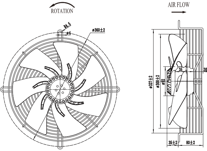
■ 外观尺寸 (mm) Dimensions (mm)
