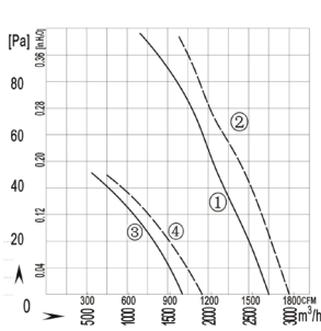
P-Q曲线 P-Q Curve
