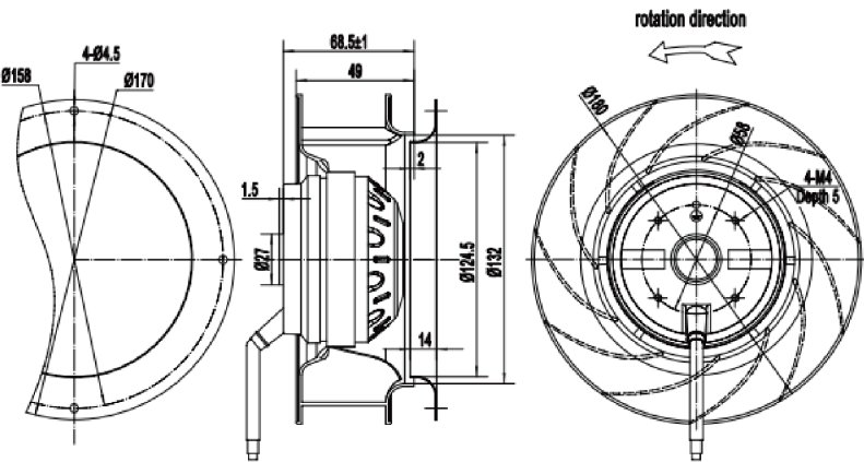
■ 外观尺寸 (mm) Dimensions (mm)
