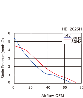
■ P-Q曲线 P-Q Curve
