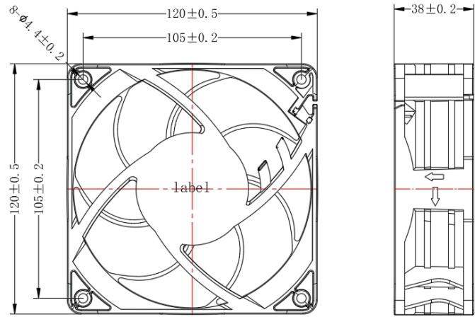
■ 外观尺寸 (mm) Dimensions (mm)
