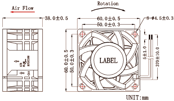
■ 外观尺寸 (mm) Dimensions (mm)
