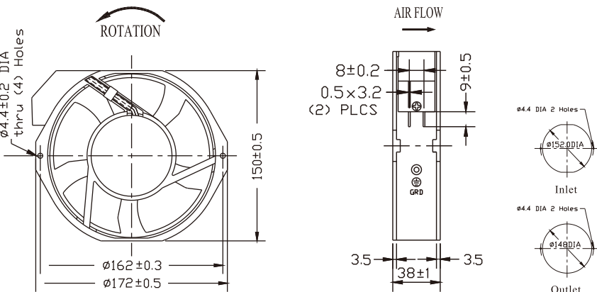
■ 外观尺寸 (mm) Dimensions (mm)
