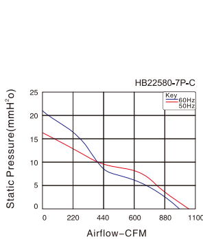
■ P-Q曲线 P-Q Curve
