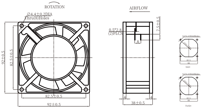
■ 外观尺寸 (mm) Dimensions (mm)
