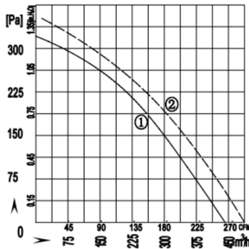
■ P-Q曲线 P-Q Curve
