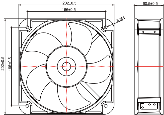
■ 外观尺寸 (mm) Dimensions (mm)
