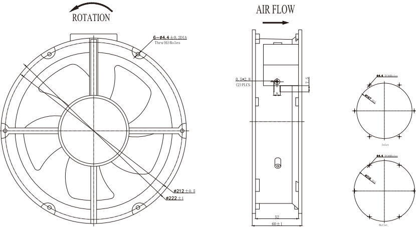
■ 外观尺寸 (mm) Dimensions (mm)
