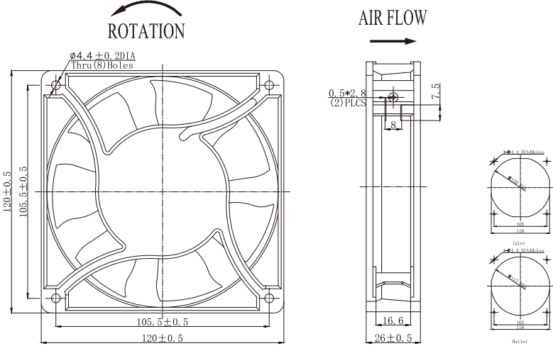
■ 外观尺寸 (mm) Dimensions (mm)
