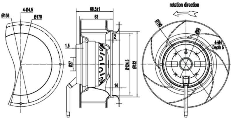
■ 外观尺寸 (mm) Dimensions (mm)
