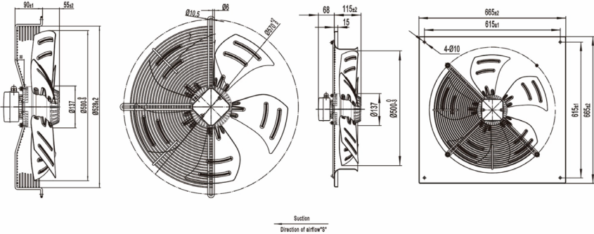
■ 外观尺寸 (mm) Dimensions (mm)
