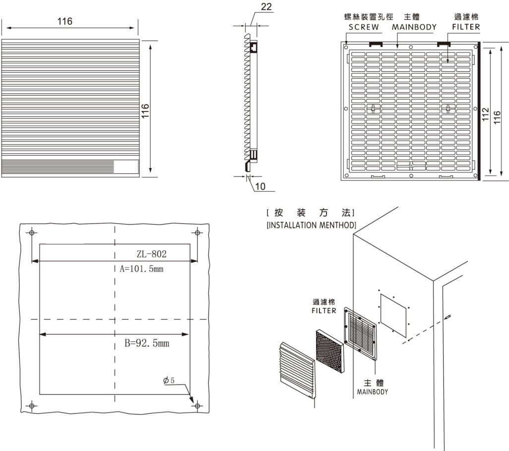
■ 使用安装方法 Use the installation method
