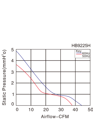
■ P-Q曲线 P-Q Curve
