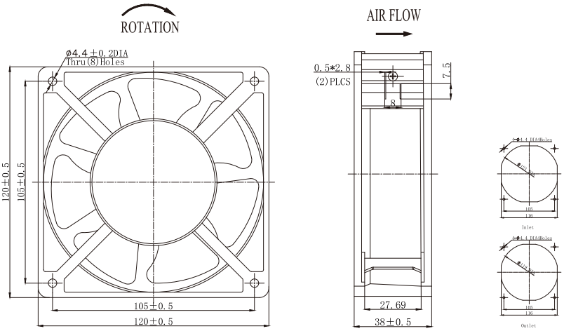
■ 外观尺寸 (mm) Dimensions (mm)
