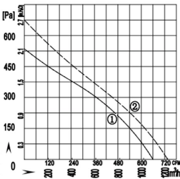
■ P-Q曲线 P-Q Curve
