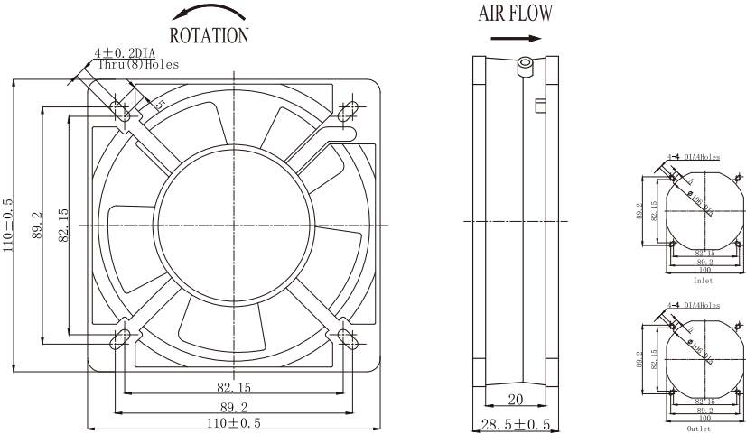
■ 外观尺寸 (mm) Dimensions (mm)
