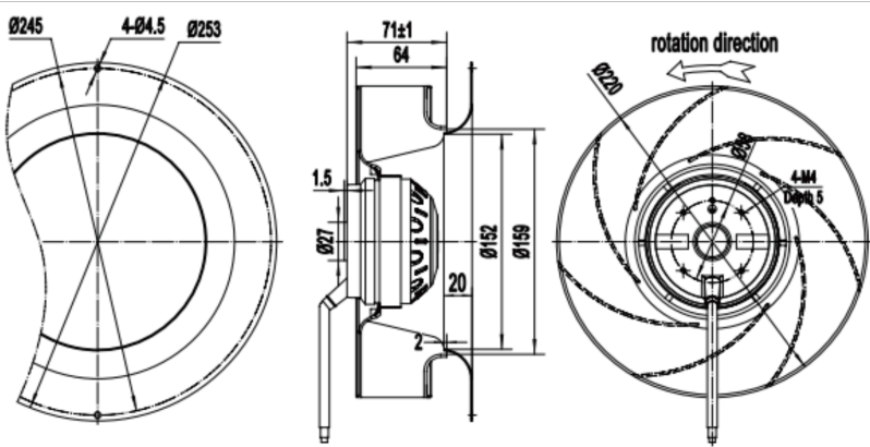
■ 外观尺寸 (mm) Dimensions (mm)
