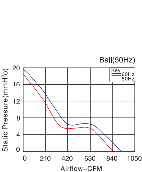
■ P-Q曲线 P-Q Curve
