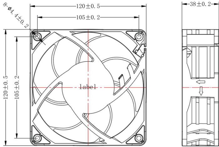
外观尺寸 (mm) Dimensions (mm)
