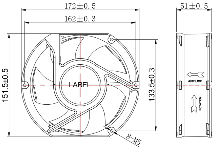
■ 外观尺寸 (mm) Dimensions (mm)
