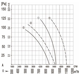
P-Q曲线 P-Q Curve
