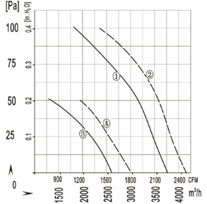
P-Q曲线 P-Q Curve
