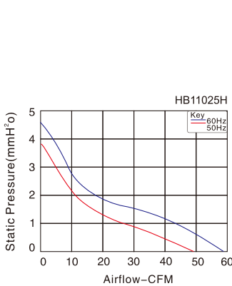
■ P-Q曲线 P-Q Curve
