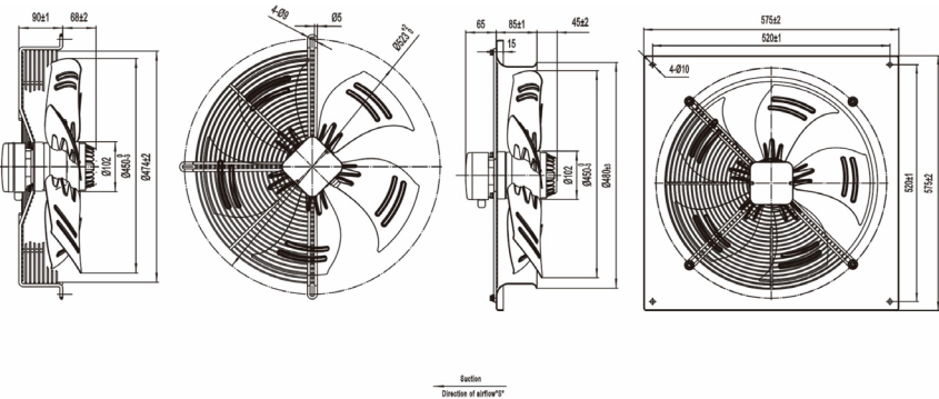
■ 外观尺寸 (mm) Dimensions (mm)
