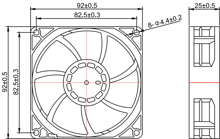
外观尺寸 (mm) Dimensions (mm)
