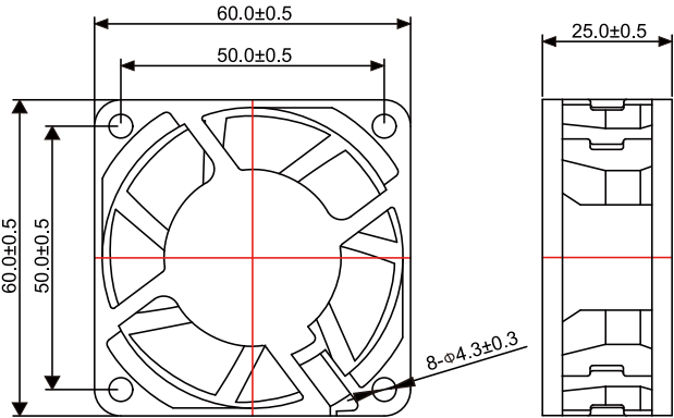
■ 外观尺寸 (mm) Dimensions (mm)
