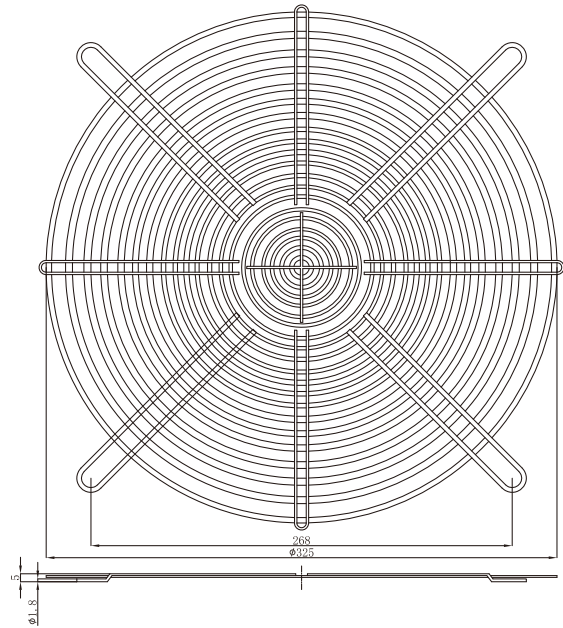
▪ JL-300 For 300mm Fan
