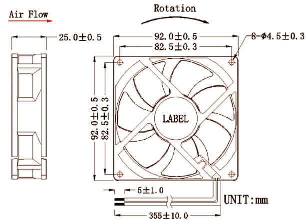
外观尺寸 (mm) Dimensions (mm)
