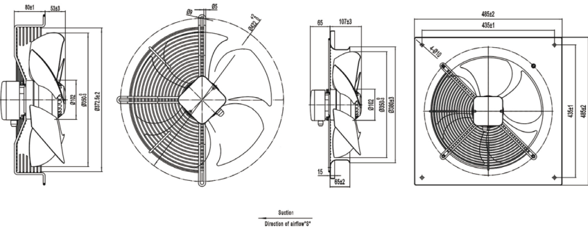
外观尺寸 (mm) Dimensions (mm)
