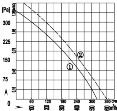
■ P-Q曲线 P-Q Curve
